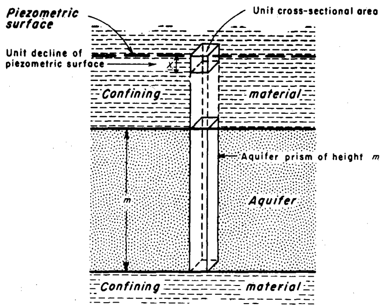
A. ARTESIAN AQUIFER
